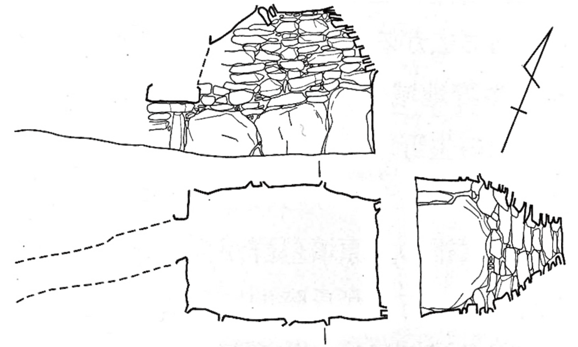
宫山古坟石室测量图
