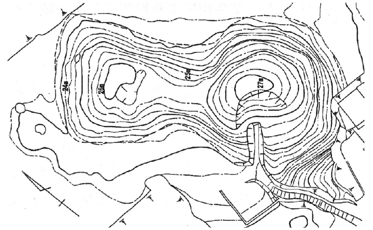
宫山古坟坟丘测量图 古墳墳丘測量図
